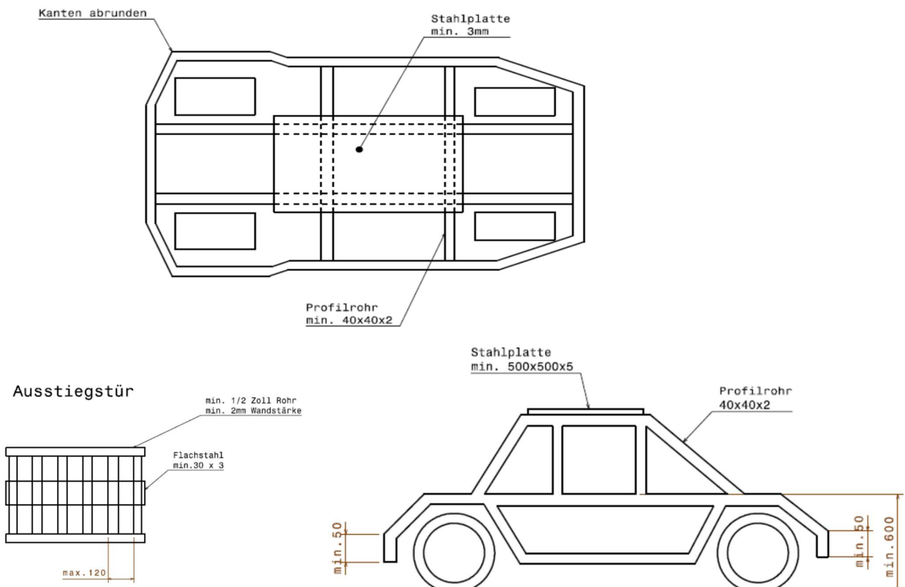
Aufbau Bodenplatte
