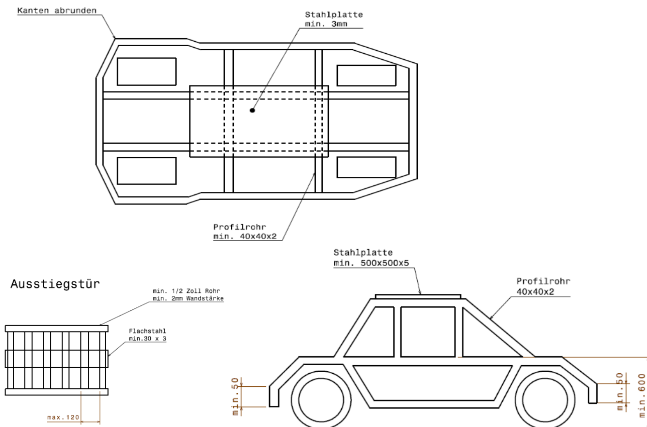
Aufbau Bodenplatte
